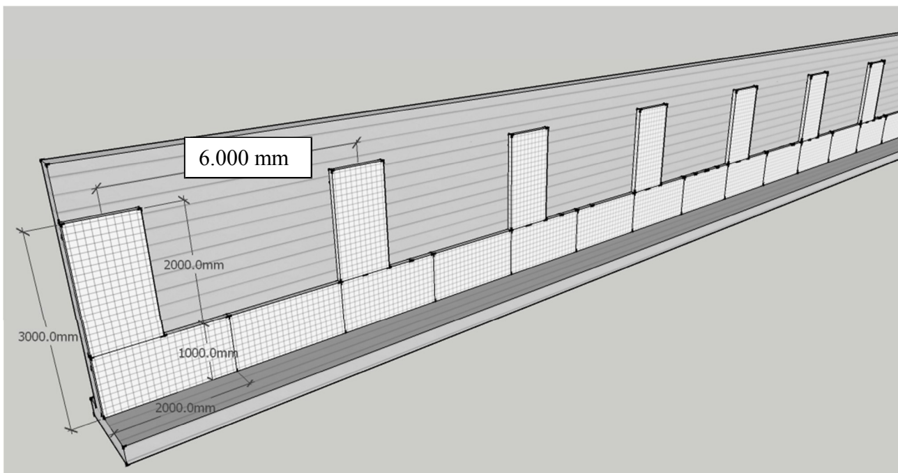
Abb. 1. Anordnung als Drainagesäulen H=2, Abstand 6 m
