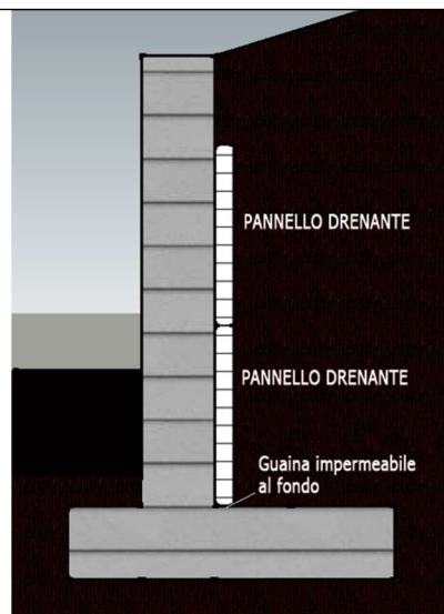
SISTEMA DE PANELES DRENANTES
