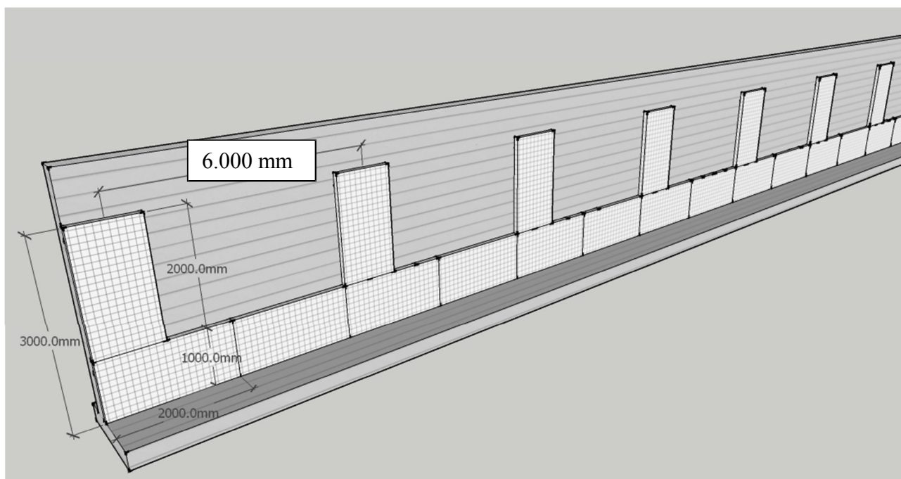
Fig. 1. Disposición en pilares drenantes H=2, distancia entre ejes de 6 m
